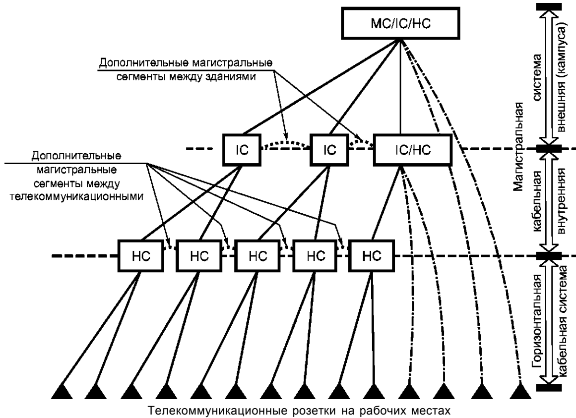
Рисунок 24 — Дополнения к базовой топологии типа «звезда» магистральной кабельной подсистемы
