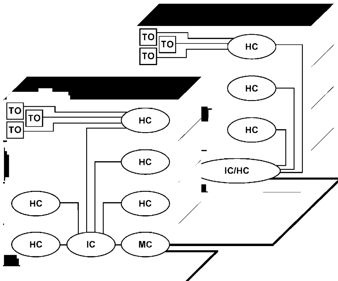
Рисунок 8 — Кабельная система с кроссами, выполняющими комбинированные функции (1С/НС во втором здании)
