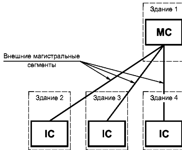
Рисунок 25 — Внешняя магистральная кабельная подсистема (магистральная подсистема кампуса)
